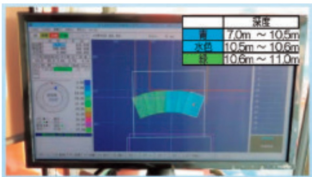
浚渫管理システムによる浚渫工の可視化
