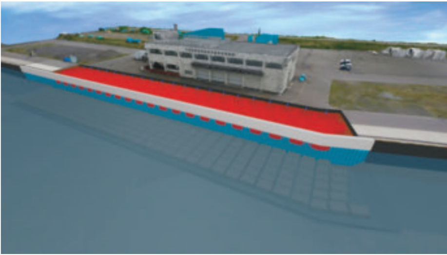
【3D モデル】 設計図面から BIM/CIM モデル（ドローン映像との組合せ）
