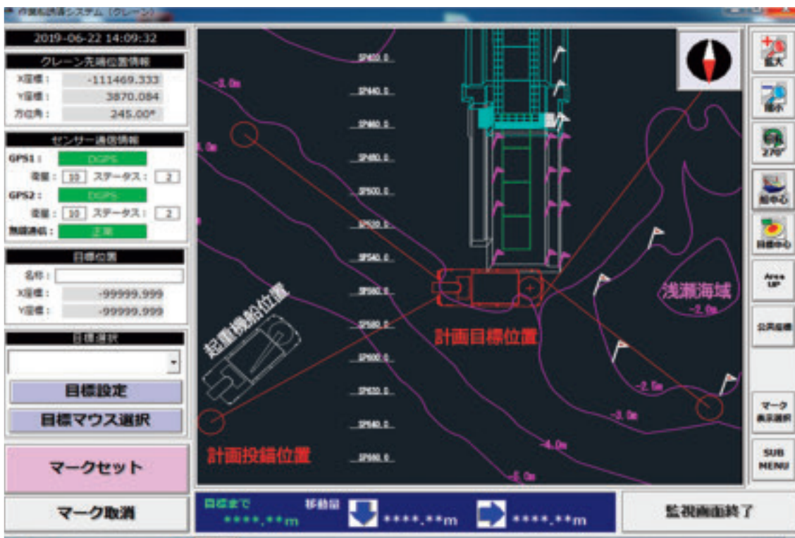
GNSS による作業船位置誘導管理システム (捨石投入時の起重機船投錨作業)
