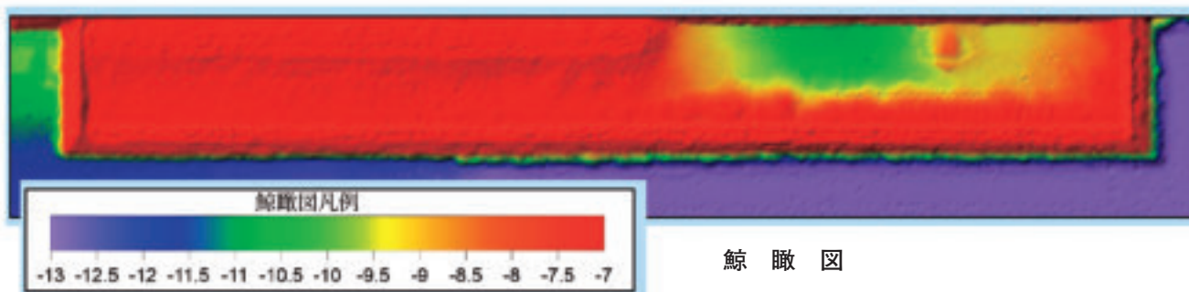
マルチビーム音響測深機による土捨工の可視化
