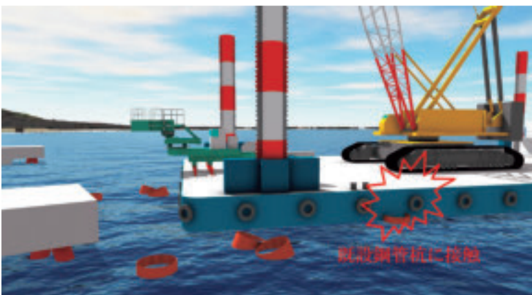
施工時のリスク評価
