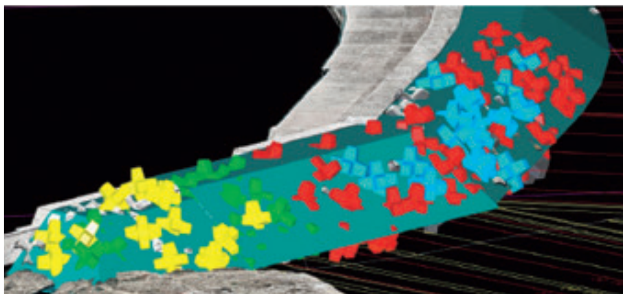
消波ブロックの据付シミュレーション
